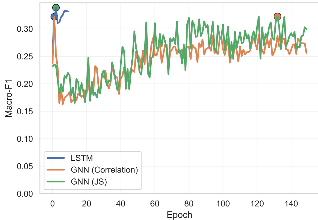
Validation macro-F1
